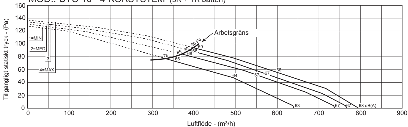
MOD.: UTC 20 - 4-RÖRSYSTEM (3R + 1R batteri)
