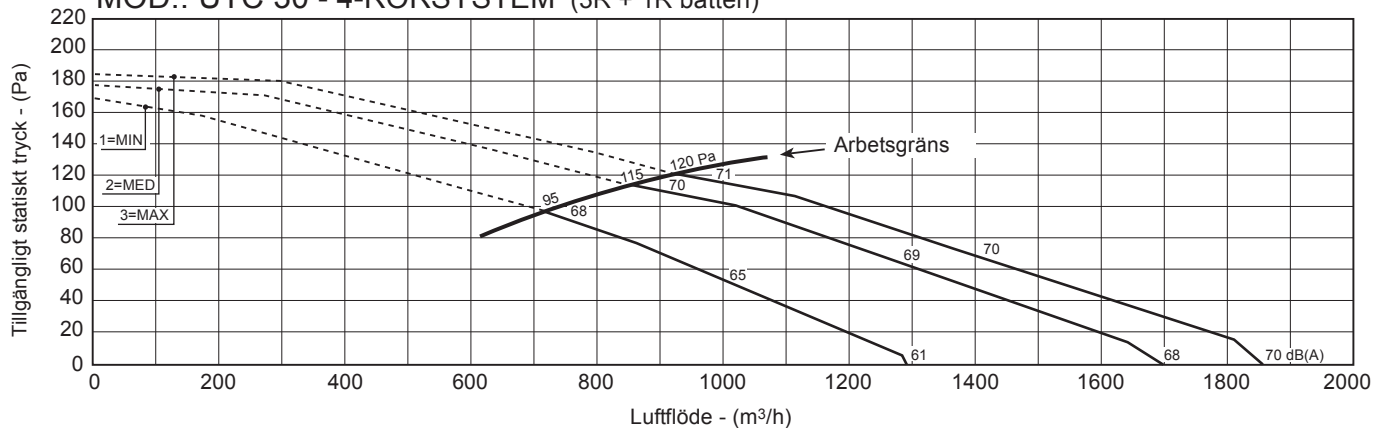
MOD.: UTC 30 - 4-RÖRSYSTEM (3R + 1R batteri)
