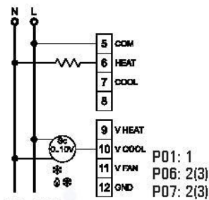
Fig. 12f. Elvärmsystem med 0 ... 10V servokontroll
