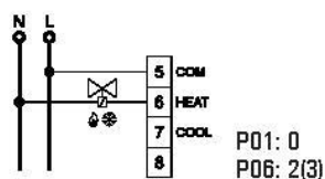
Fig. 12a. 2-rörssystem med ON/OFF ventil
