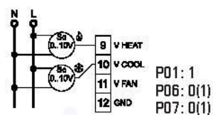
Fig. 12d. 4-rörssystem med två 0 ... 10V servokontroller
