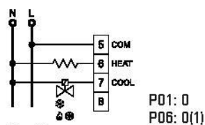
Fig. 12e. Elvärmsystem med ON/OFF ventil
