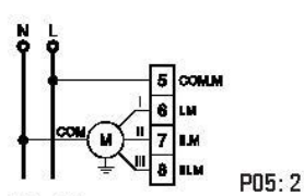
Fig. 13b. Anslutning av fläkt med 3-hastighetsmotor
