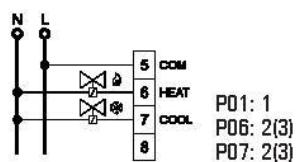
Fig. 12c. 4-rörssystem med två ON/OFF ventiler
