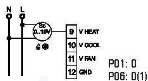
Fig. 12b. 2-rörssystem med 0 ... 10V servokontroll
