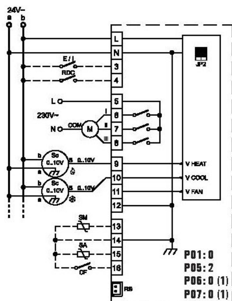
Fig. 10: Elschema för 2st 0 ... 10V, 24V ställdon i 4-rörssystem och 3-hastighets fläktmotor
