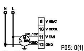
Fig. 13a. Anslutning proportionell fläkt med EC motor och 0 ... 10V ingång
