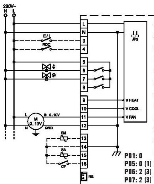
Fig. 8: Elschema för 2 on/off 230V ställdon i 4-rörssystem samt proportionell fläktdrift
