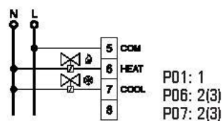
Fig. 12c. 4-rörssystem med två ON/OFF ventiler
