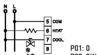
Fig. 12e. Elvärmesystem med ON/OFF ventil
