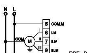
Fig. 13b. Anslutning av fläkt med 3-hastighetsmotor
