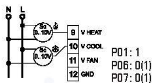
Fig. 12d. 4-rörssystem med två 0 ... 10V servokontroller
