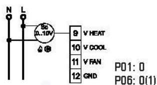
Fig. 12b. 2-rörssystem med 0 ... 10V servokontroll
