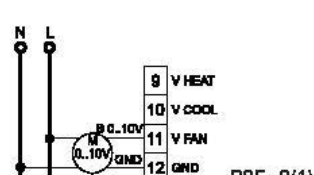
Fig. 13a. Anslutning proportionell fläkt med EC motor och 0 ... 10V ingång
