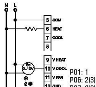
Fig. 12f. Elvärmesystem med 0 ... 10V servokontroll
